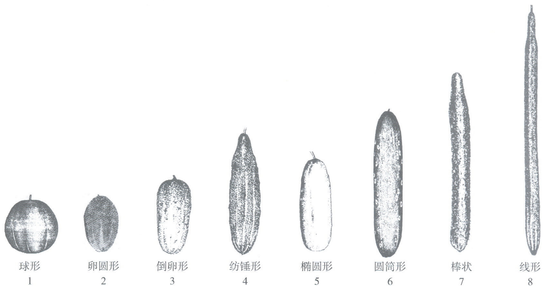
图 B.4 果实:形状
