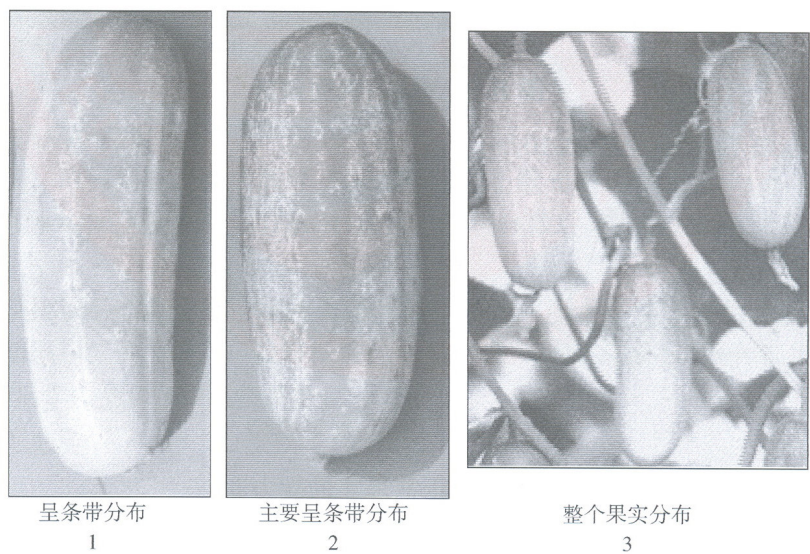
图 B. 7 果实:表面斑块分布
