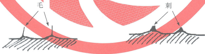
图 B.10 果实:刺毛类型
