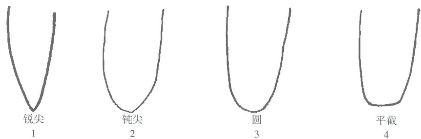
图 B. 5 果实:顶部形状
