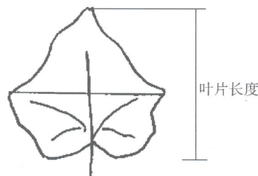
图 B.3 叶片:长度
