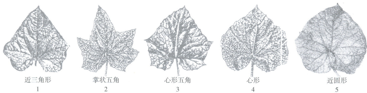
图 B.1 叶片:形状
